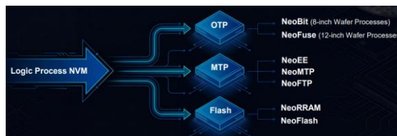
圖一、邏輯製程非揮發性記憶體
